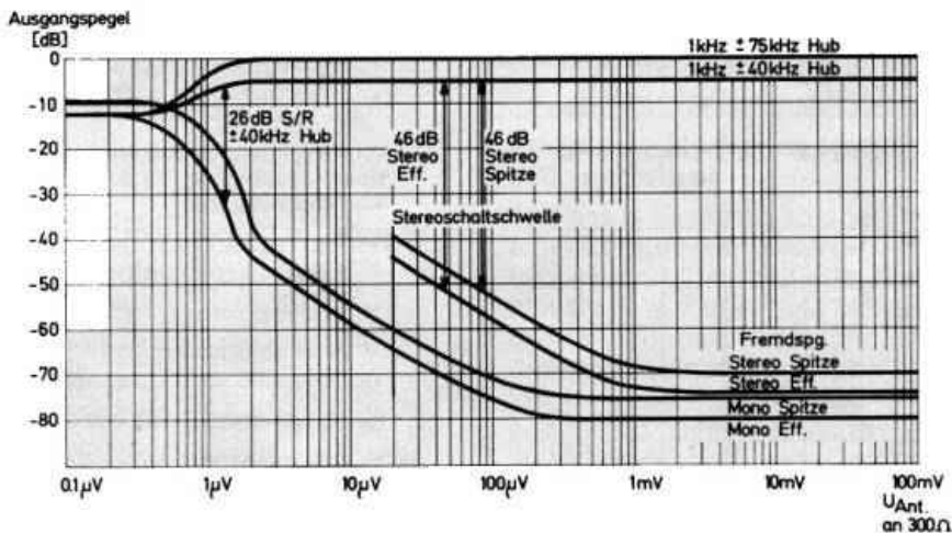
Fremdspannungsabstand FM in Abhängigkeit von der Antennenspannung.
