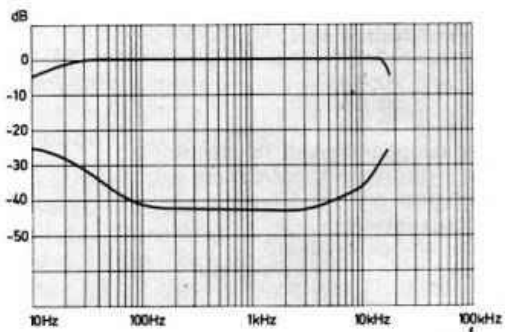
Obersprechdämpfung UKW-Stereo, 100 MHz, 1 mV HF-Pegel an 75-Ω-Antenneneingang, gemessen am Lautsprecherausgang.
