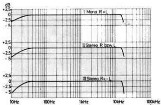
Frequenzgang FM-Mono/Stereo von Antenne bis Lautsprecherausgang (1 mV HF-Pegel an 75 Ω/100 MHz).
