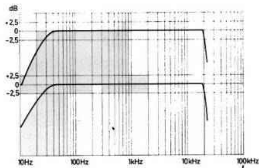
Frequenzgang TA-Magnet (über Schneidkennlinien-Nachbildung) mit steilem Abfall der Frequenzen unterhalb 40 Hz, gemessen am Lautsprecherausgang.
