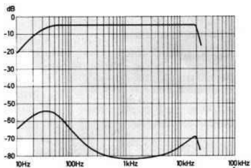
Obersprechdämpfung L→R/R→L, gemessen über Schneidkennlinien-Nachbildung (Meßeingang TA-Magnet).
