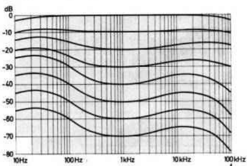
Verlauf der gehörrichtigen Lautstärkekorrektur (Contour).
